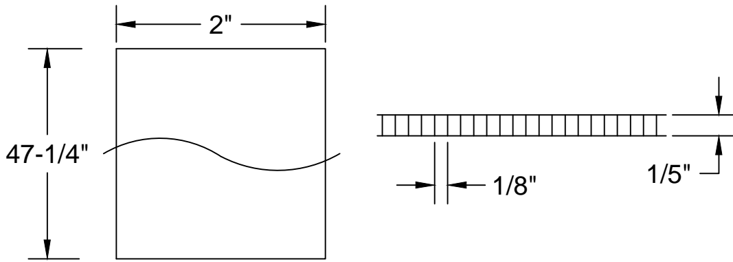
5mm SPACER (FS1005)
